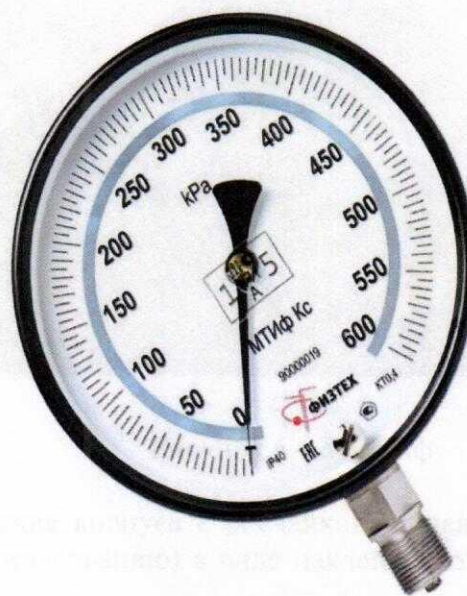
Рисунок 2 – МТФ Кс
